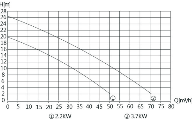
性能曲线图
