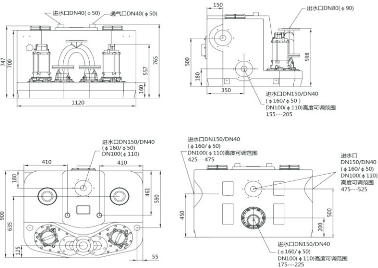
设备尺寸图
