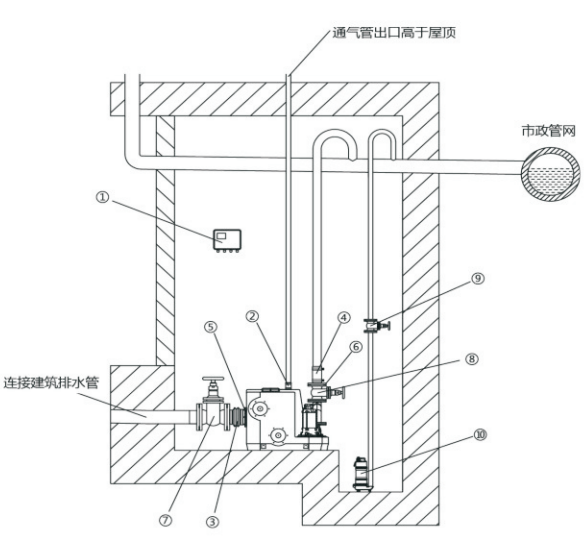
安装示意图
